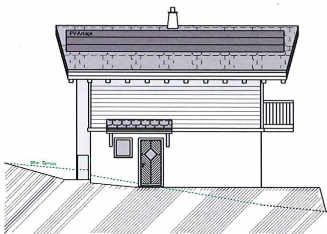
ANSICHT OST
