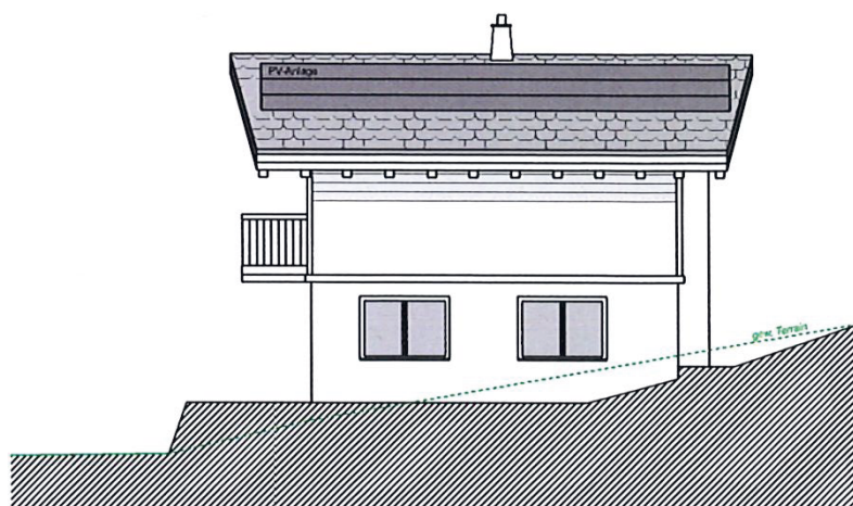
ANSICHT WEST
