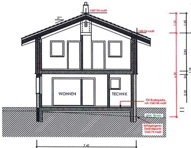
GEBÄUDESCHNITT A - A 1:100 HAUS A
