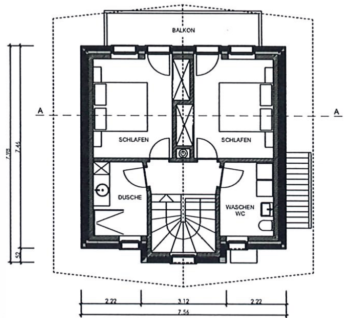
GRUNDRISS OBERGESCHOSS 1:100
