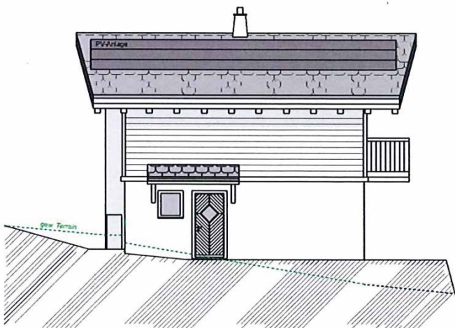
ANSICHT OST
