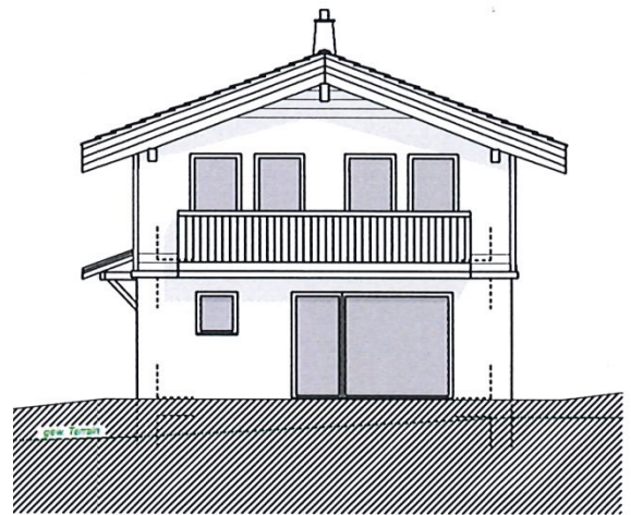
ANSICHT NORD
