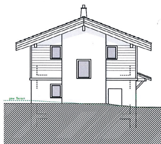
ANSICHT SÜD
