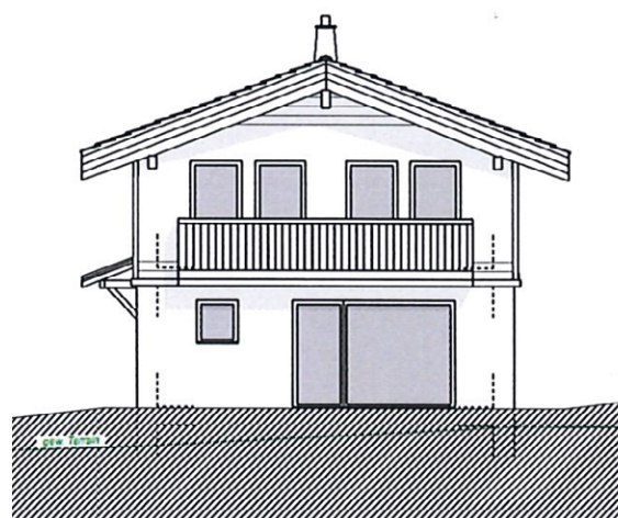
ANSICHT NORD
