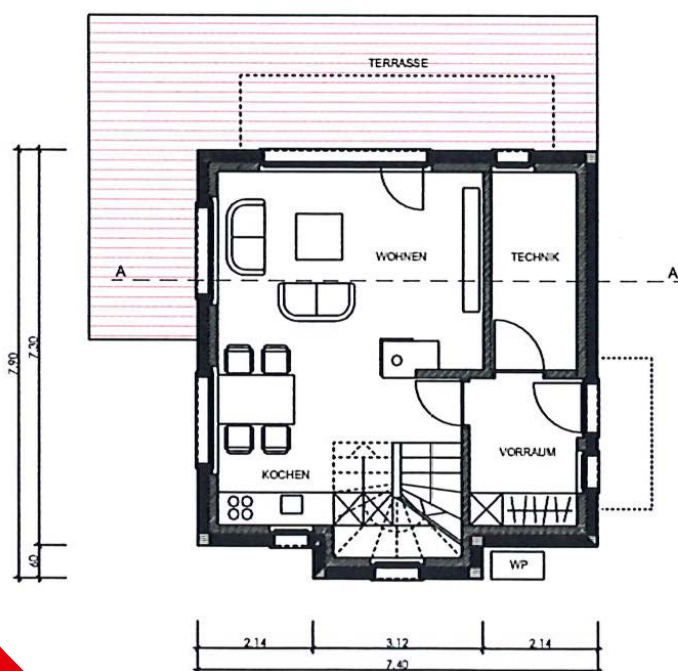
GRUNDRISS ERDGESCHOSS 1:100
