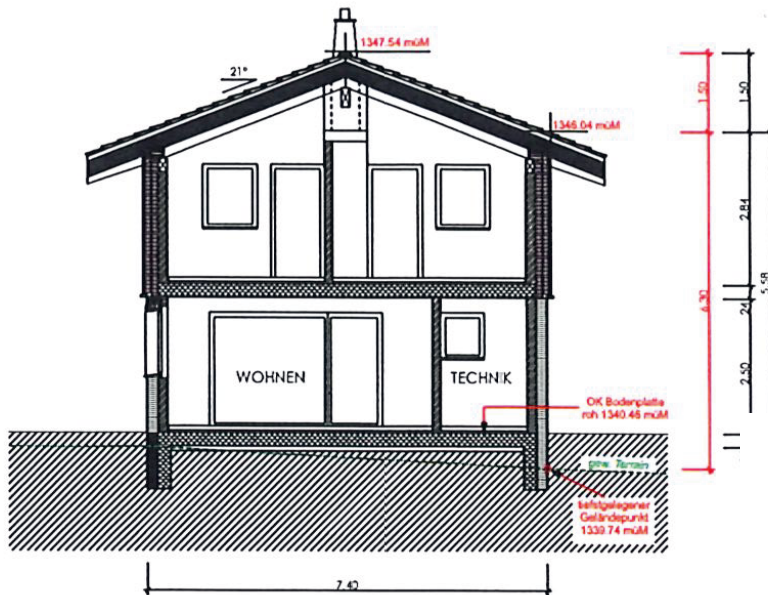
GEBÄUDESCHNITT A - A 1:100
