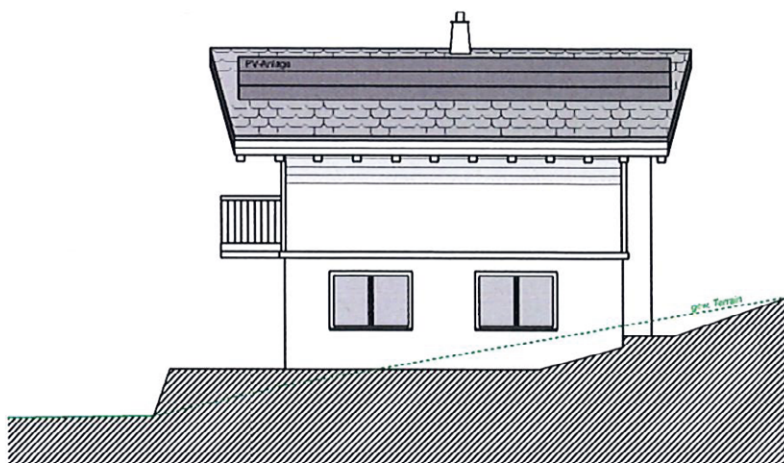
ANSICHT WEST
