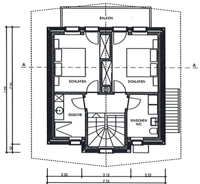
GRUNDRISS OBERGESCHOSS 1:100
